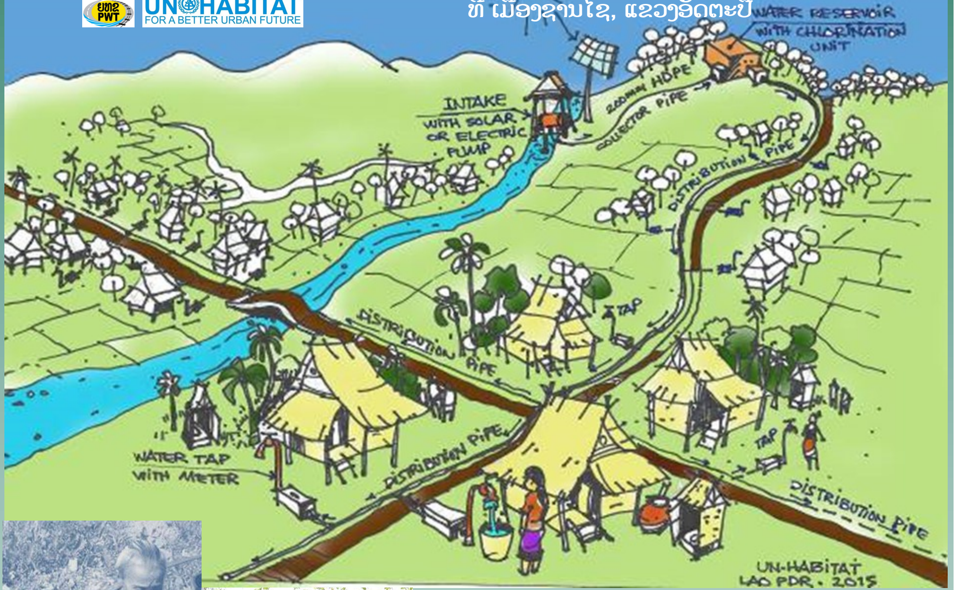
ຮູບທັດສະຍະພາບ ລະບົບນໍ້າປະປາຂະໜາດນ້ອຍ
