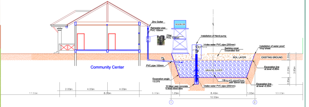
ແບບ ຮູບຕັດອ່າງເກັບນໍ້າຝົນໄຕ້ດິນ
